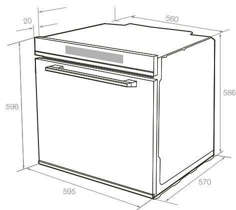
Encastre en Mueble Built in Dimensions
